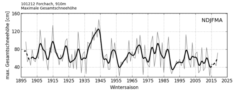
maximale Gesamtschneehöhe
