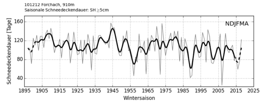
Schneedeckendauer
