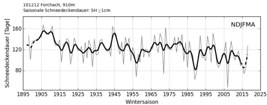
Schneedeckendauer
