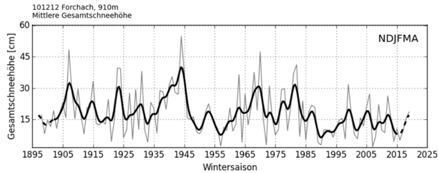
mittlere Gesamtschneehöhe
