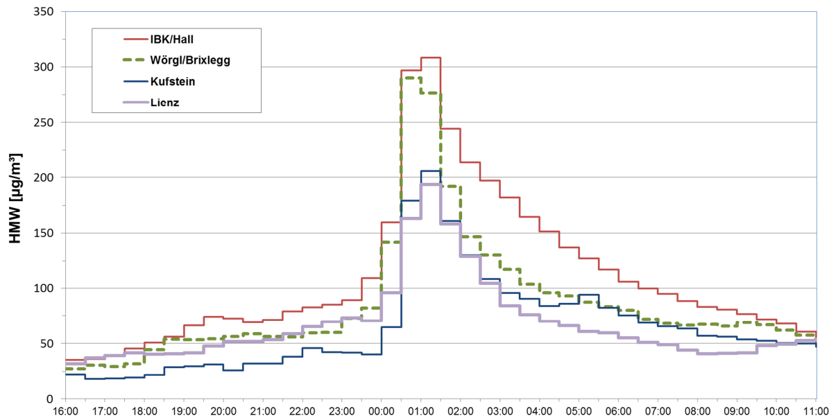
Abbildung 1: Durchschnittliche Halbstundenmittelwerte (HMWe) der PM10-Feinstaubkonzentration in der Silvesternacht ermittelt an den Messstellen in städtischen Gebieten. Die Werte präsentieren die Durchschnittswerte jeweils am 31.12.(2010-2017) und am 1.1.(2011-2018).
