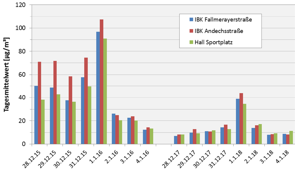
Abbildung 4: Tagesmittelwerte der PM10-Feinstaubbelastung an den Messstellen Innsbruck/Fallmerayerstraße, Innsbruck/Andechsstraße und Hall/Sportplatz (Ballungsraum Innsbruck/Hall) an den Tagen um den Jahreswechsel 2015/16 und 2017/18. Ein Föhneinbruch zu Jahresbeginn 2016 führte zu einer raschen Abnahme der Feinstaubbelastung an den drei Messstationen während dichter Nebel die Feinstaubkonzentrationen 2017/18 deutlich reduzierte (vgl. Abbildung 2 und 3).
