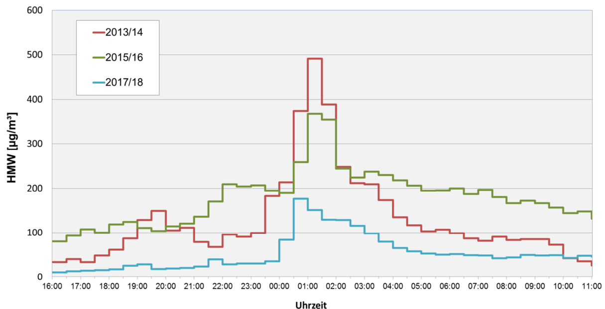
Abbildung 3: Verlauf der Feinstaubbelastung PM 10 an der Messstation Innsbruck/Andechsstraße während drei Silvesternächten mit unterschiedlichen Witterungseinflüssen (rot = labile Witterungsverhältnisse, grün = Inversionswetterlage; blau = Inversionswetterlage mit starkem Nebel). HMW = Halbstundenmittelwert.
