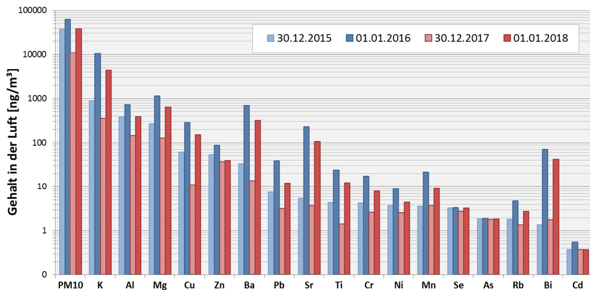
Abbildung 5: Mittlere Gehalte an PM10 und den darin enthaltenen Metallen in der Luft jeweils am 30.12. und am Neujahrstag 2015/16 und 2017/18 im Ballungsraum Innsbruck/Hall. Der 30.12. kann als Hintergrundbelastung ohne (bzw. mit geringem) Feuerwerkseinfluss angenommen werden. (PM10 = Feinstaub in der Atemluft mit einem aerodynamischen Durchmesser von \leq 10 \mu\text{m} ). Die logarithmische Skalierung der Vertikalachse ist zu beachten.
