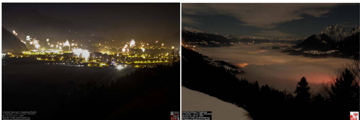
Abbildung 2: Feuerwerke zum Jahreswechsel im Inntal bei unterschiedlichen Witterungsbedingungen; linkes Bild: 1.1.2017 um 00:12 Uhr (Webkamera der Abt. Waldschutz am Standort Kramsach/Angerberg); rechtes Bild: Starker Nebel am Talboden am 1.1.2018 um 00:12 Uhr (Webkamera der Abt. Waldschutz am Standort Schwaz/Kogelmoos).
