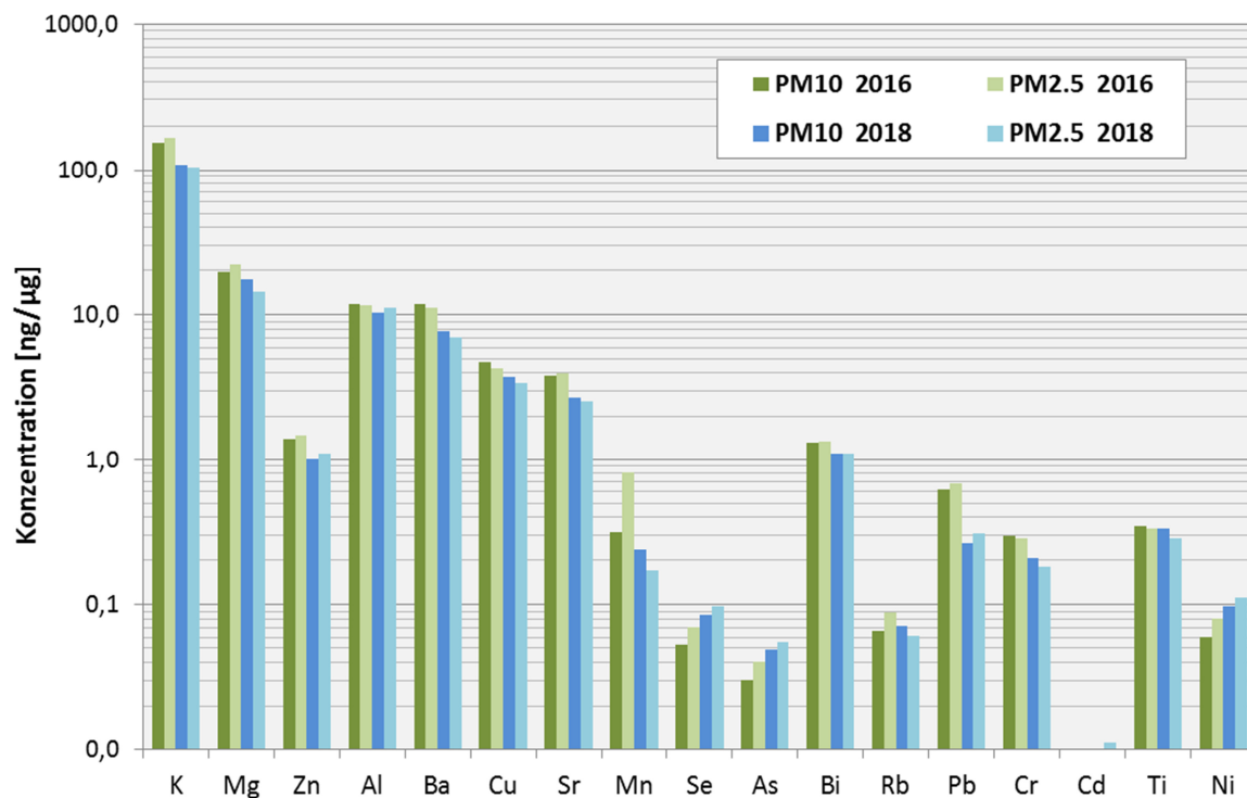
Abbildung 7: Gehalte an Metallen in den Feinstäuben PM10 und PM2.5 an den Neujahrstagen 2016 und 2018 an der Messstelle Innsbruck/Fallmerayerstraße. Man beachte die logarithmische Skalierung der Vertikalachse.
