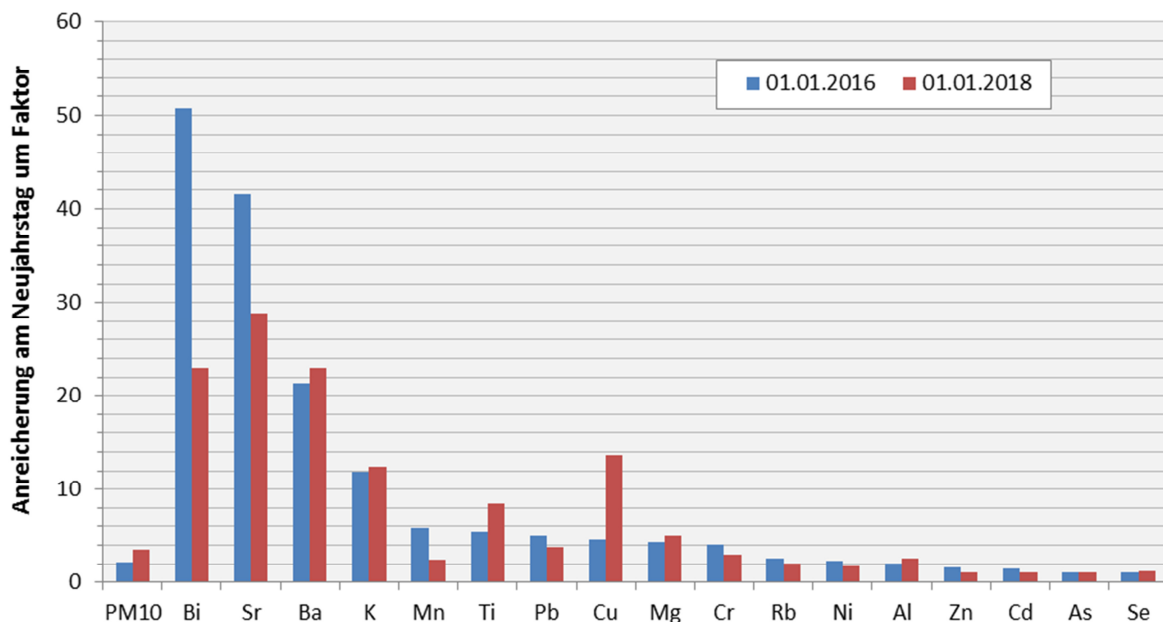
Abbildung 6: Durchschnittliche Anreicherung von PM10 und den darin enthaltenen Metallen in der Luft an den Neujahrstagen im Vergleich zum 30.12. des jeweiligen Vorjahrs im Ballungsraum Innsbruck/Hall.
