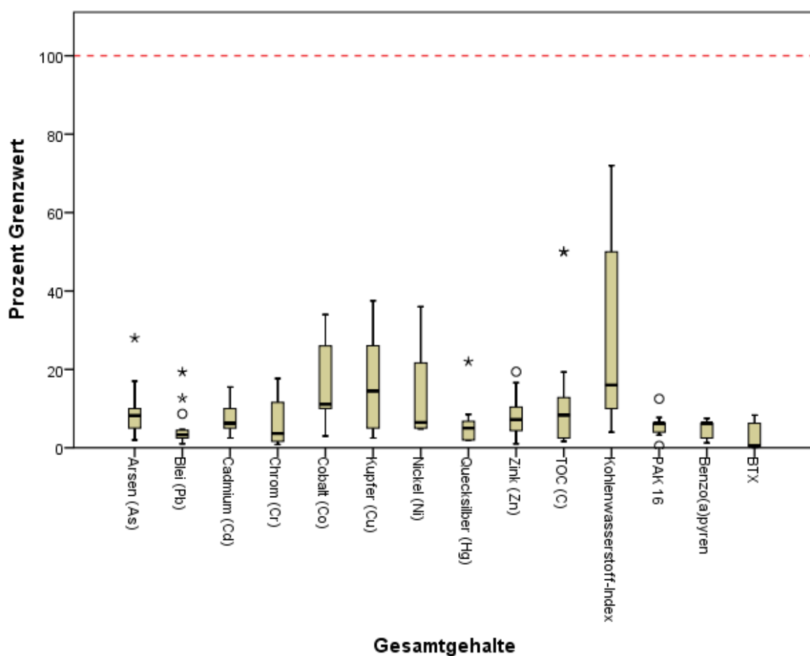
Abb. 13-1: Analyseergebnisse in % der Grenzwerte der Bodenaushubdeponie (DVO 2008 Anhang 1, Tab.1, Spalte I)
