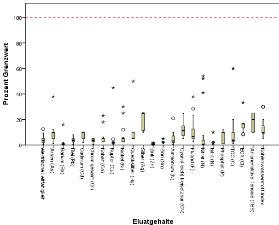
Abb. 13-2: Analyseergebnisse in % der Grenzwerte der Bodenaushubdeponie (DVO 2008 Anhang 1, Tab.2)
